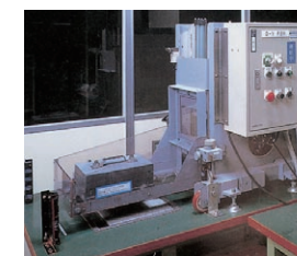
施工例：IPF-300/GRL-12
